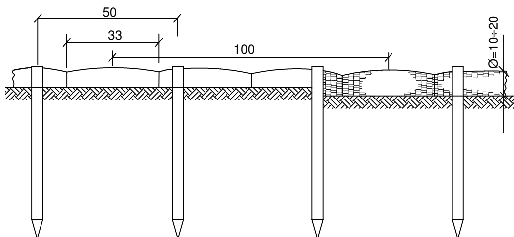
Przekrój podłużny
